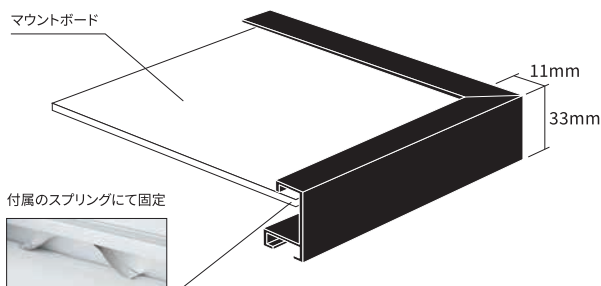
フレーム断面図
